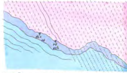
Fig. 6. Überspringen der Gneisschieferung auf den Kalk am Mettenberg ( obere Contactlinie )
